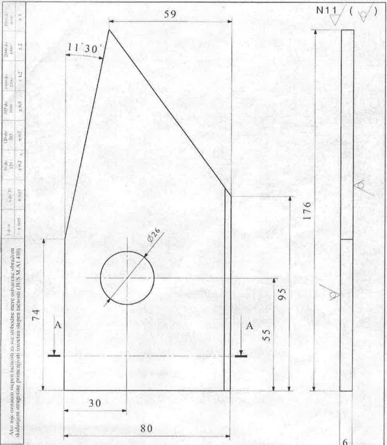
Presek "A-A"
