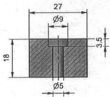
A-A (1:1)
