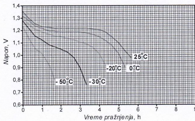
Sl.2 Krive pražnjenja Ni-Cd akumulatora, tip KPM-60P sa konstantnom strujom 0,2 C 5 (A), na razlicitim temperaturama okoline
