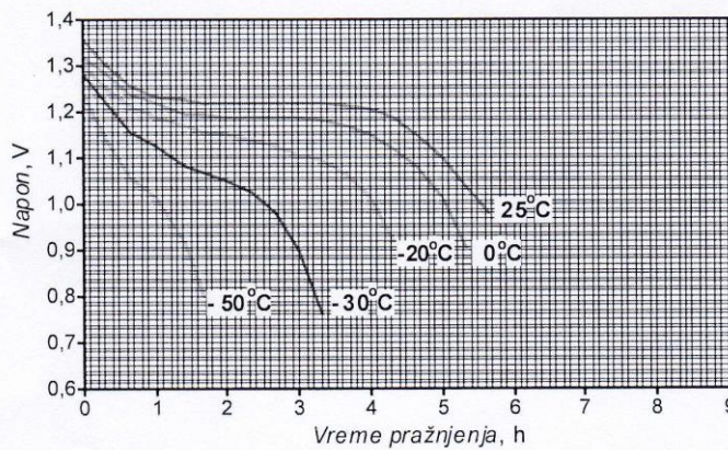
SI.2 Krive pražnjenja Ni-Cd akumulatora, tip KPM-120P sa konstantnom strujom 0,2 C_5(A) , na razlicitim temperaturama okoline
