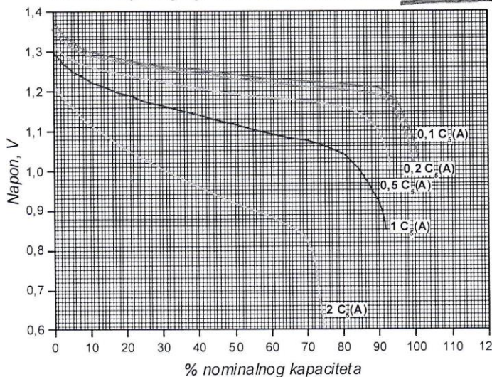
SI.3 Krive pražnjenja za Ni-Cd akumulator, tip KPM-120P
