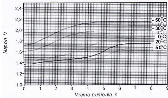
Sl.1 Krive punjenja Ni-Cd akumulatora, tip KPM-60P sa konstantnom strujom 0,2 C 5 (A), na razlicitim temperaturama okoline
