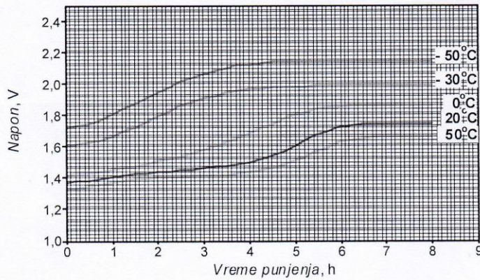
SI.1 Krive punjenja Ni-Cd akumulatora, tip KPM-120P sa konstantnom strujom 0,2 C_5(A) , na razlicitim temperaturama okoline
